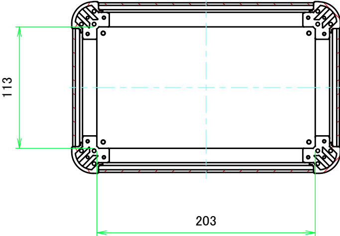
C-C ( 1 : 3.5 )
